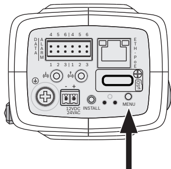
Afbeelding 6.1 Menuknop
