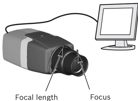
Afbeelding 6.2 Objectief instellen
