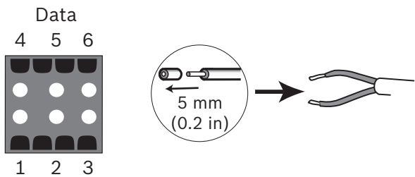
Afbeelding 5.9 Pinnen van de datastekker
