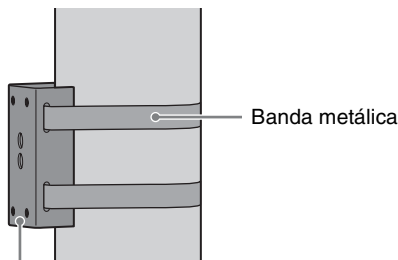
Soporte adaptador para el montaje en poste
