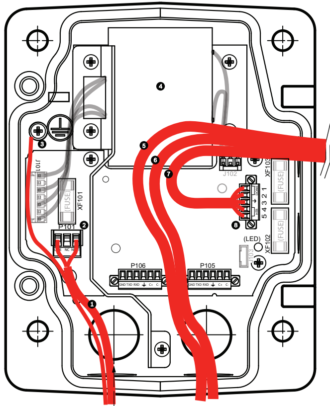
Bild 9.1: VG4-A-PSU1 oder VG4-A-PSU2 Netzteilkasten
