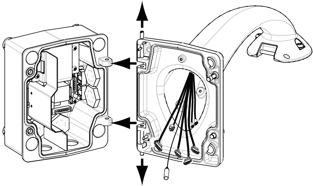
Bild 8.7: Ausrichten des Hängearms auf das Scharnier des Netzteilkastens
