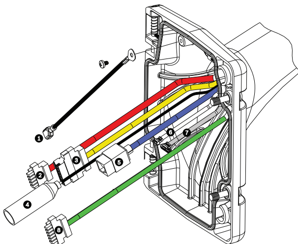
Bild 8.10: Kabel am Hängearm
