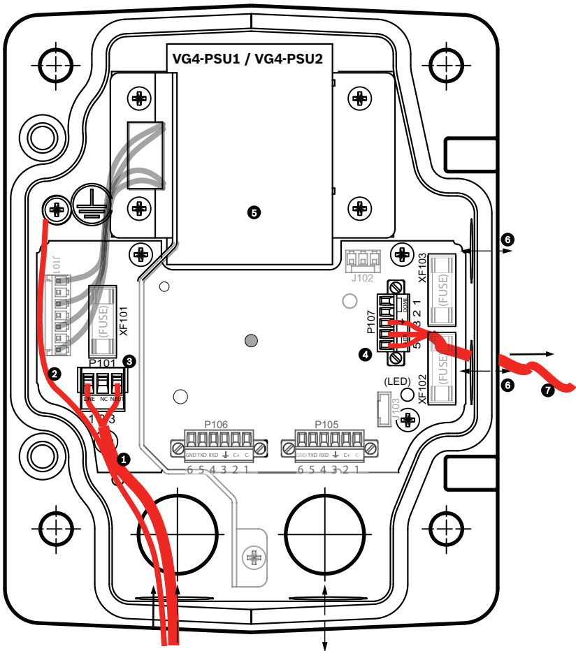
Bild 8.3: VG4-PSU1/VG4-PSU2
