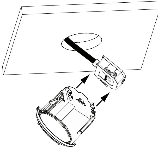
Bild 10.9: Montieren des Gehäuses an die Interface-Box
