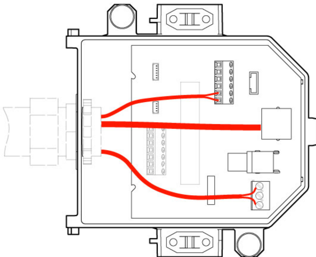
Bild 10.5: Interface-Box-Anschlüsse
