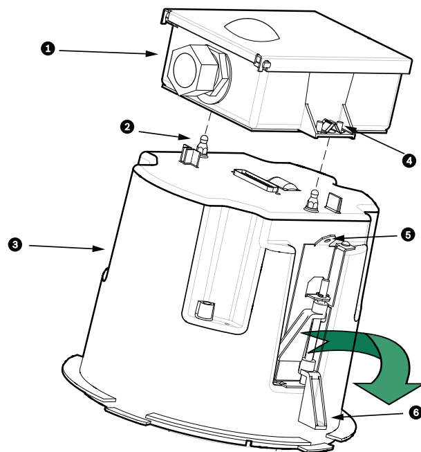
Bild 10.10: Deckeneinbaugeschoss und Interface-Box
