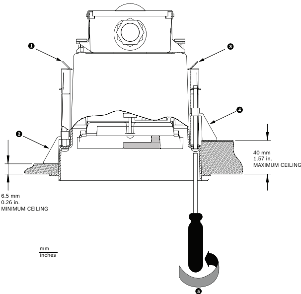
Bild 10.11: Sichern der Kamera an der Decke
