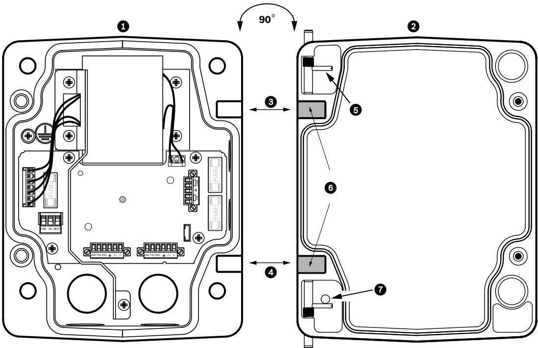
Bild 9.5: Ausrichten des Scharniers der Abdeckklappe auf den Netzteilkasten
