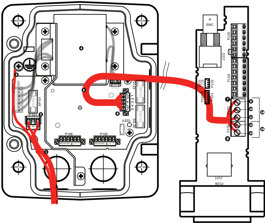
Bild 9.2: VG4-A-PSU1 oder VG4-A-PSU2 Netzteilkasten angeschlossen an die Rohrschnittstellenplatte
