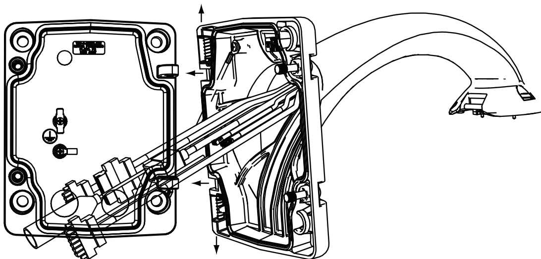
Bild 8.9: Anschließen des Hängearms an der Montageplatte
