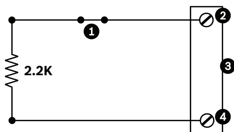
Bild 12.3: N.C.S. - Anschlüsse für überwachten Öffneralarm
