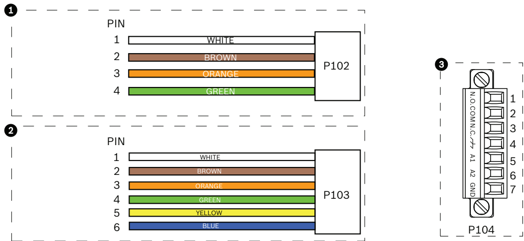
Bild 9.12: Alarm- und Relaisstecker
