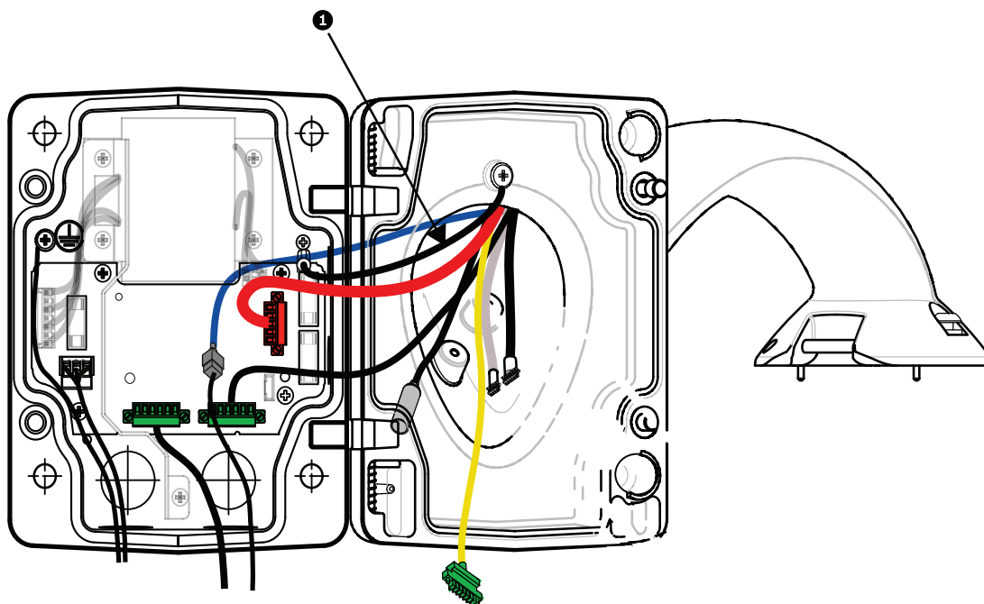
Bild 8.8: Anschließen der Hängearmleiter an den Netzteilkasten
