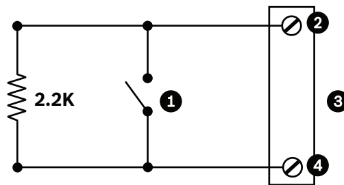
Bild 12.2: N.O.S. - Anschlüsse für überwachten Schließeralarm
