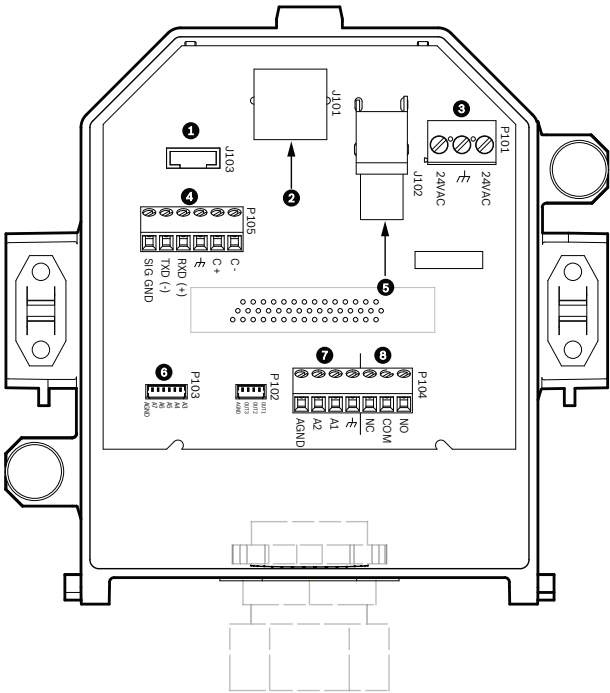
Bild 10.7: Interface-Box für den Deckeneinbau
