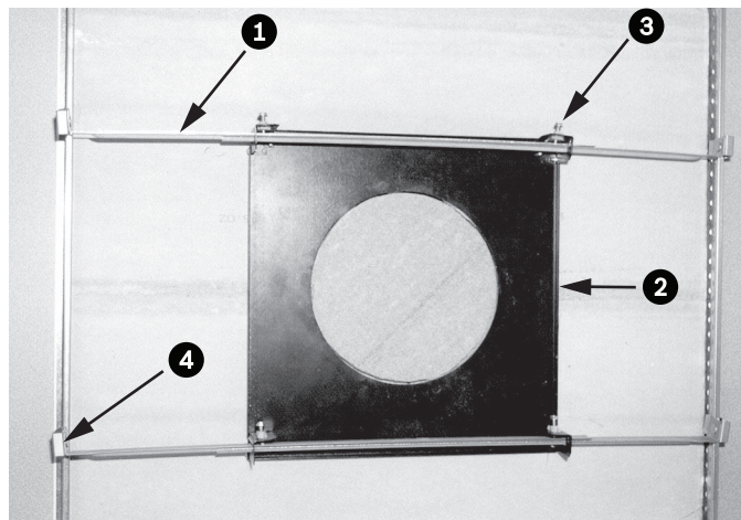
Bild 10.1: Zwischendeckenhalterung (Draufsicht)
