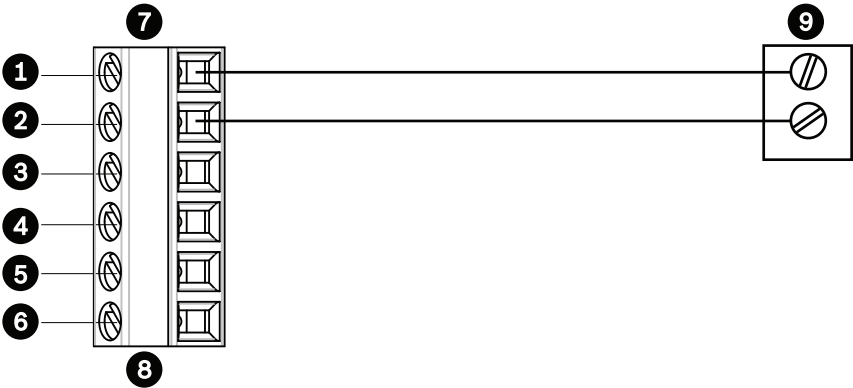
Bild 12.6: Anschlüsse für Audio über ein Ethernet-Netzwerk
