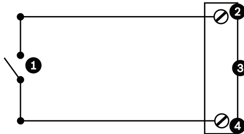
Bild 12.5: N.C. (Öffner) Anschlüsse für nicht überwachten Öffneralarm
