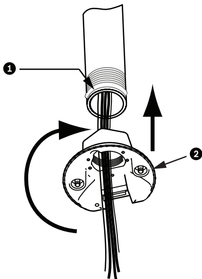
Bild 9.9: Befestigen der Dome-Kappe
