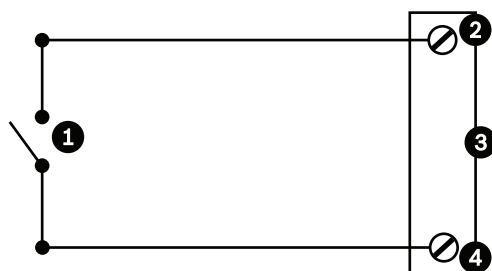
Bild 12.4: N.O. (Schließer) - Anschlüsse für nicht überwachten Schließeralarm
