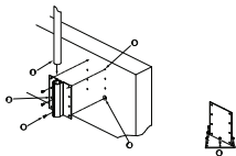
Bild 9.7: Brüstungshalterung und Dachhalterungsplatte
