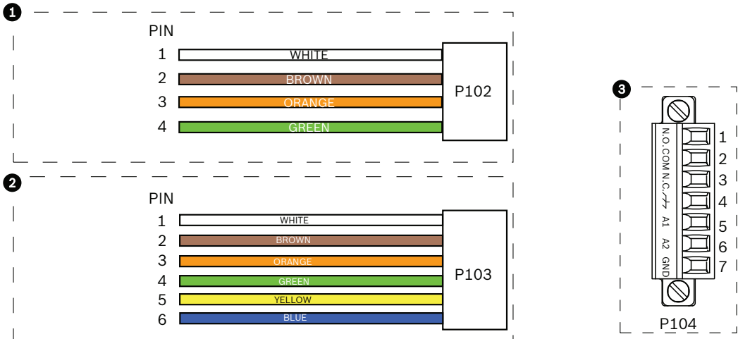
Bild 8.1: Alarm- und Relaisstecker
