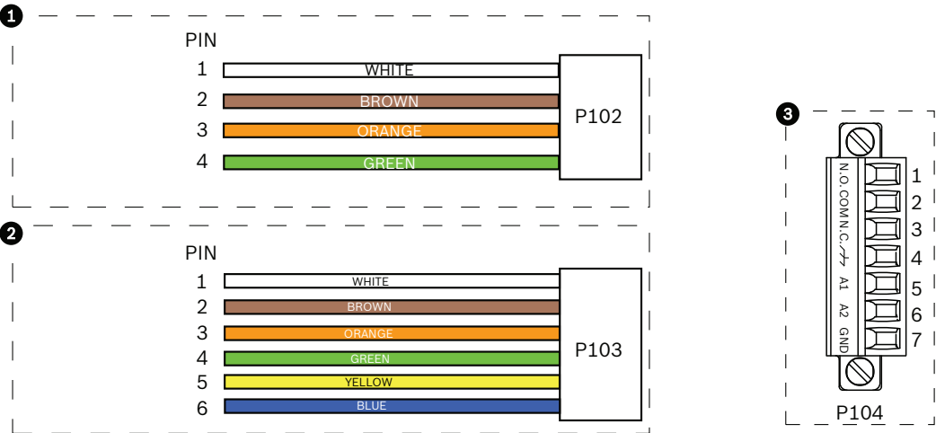
Bild 10.6: Alarm- und Relaisstecker
