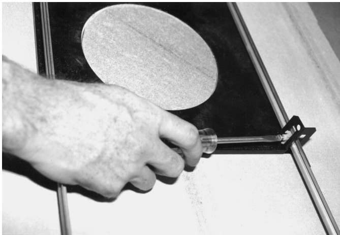
Bild 10.3: Festziehen der Sicherungsschrauben
