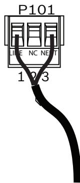
Bild 8.4: 115/230-VAC-Netzeingang
