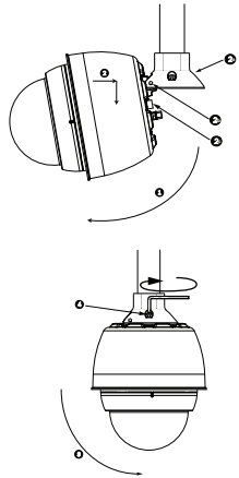
Bild 9.14: Montieren des Hängegehäuses an Dachbrüstungs-/Rohrhalterung
