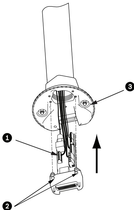
Bild 9.13: Einbauen der Rohrschnittstellenplatte in die Dome-Kappe
