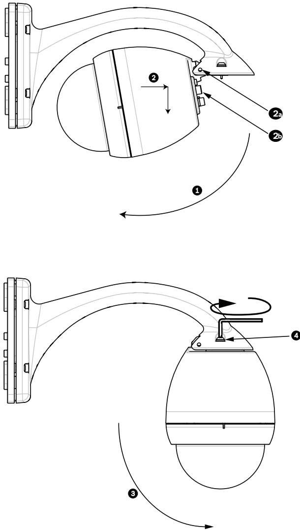
Bild 8.12: Montieren des Hängegehäuses am Arm
