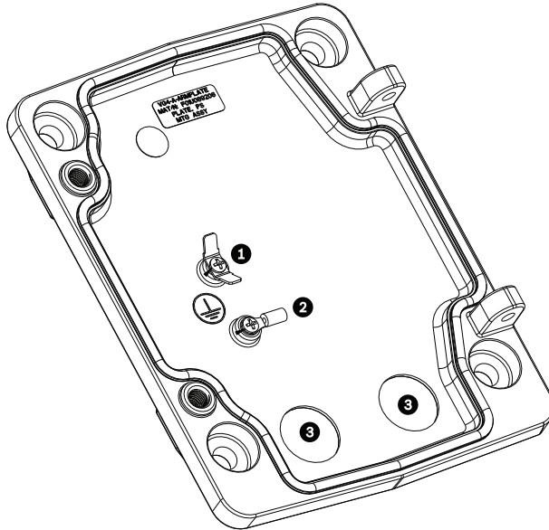
Bild 8.11: Montageplatte – Details an der Innenseite
