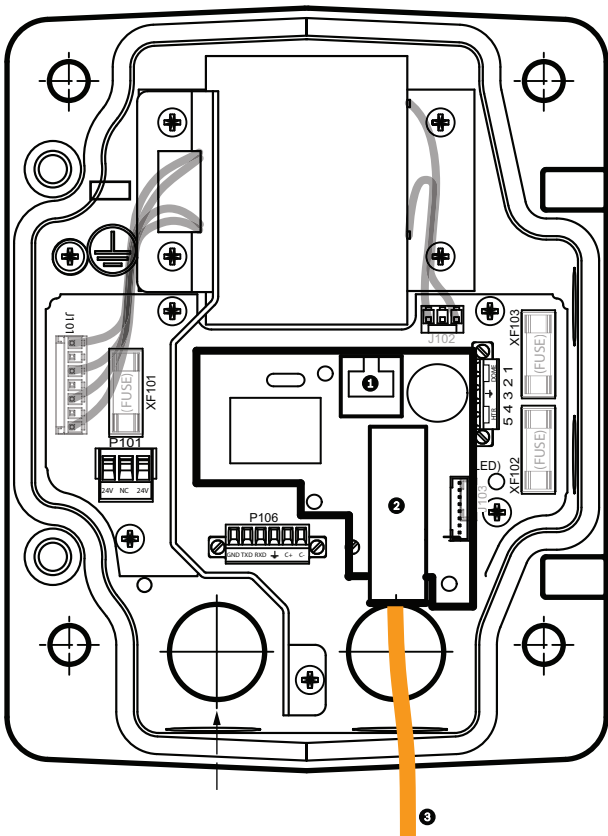
Bild 9.3: Installiertes LWL-Ethernet-Modul
