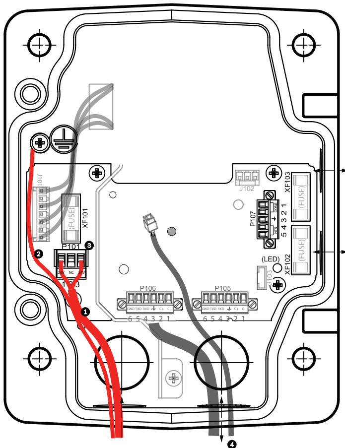
Bild 8.6: VG4-PA0 Netzteilkasten
