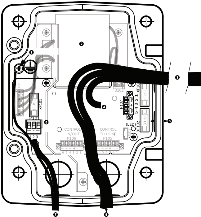
Bild 9.4: Netzteilkastenanschlüsse
