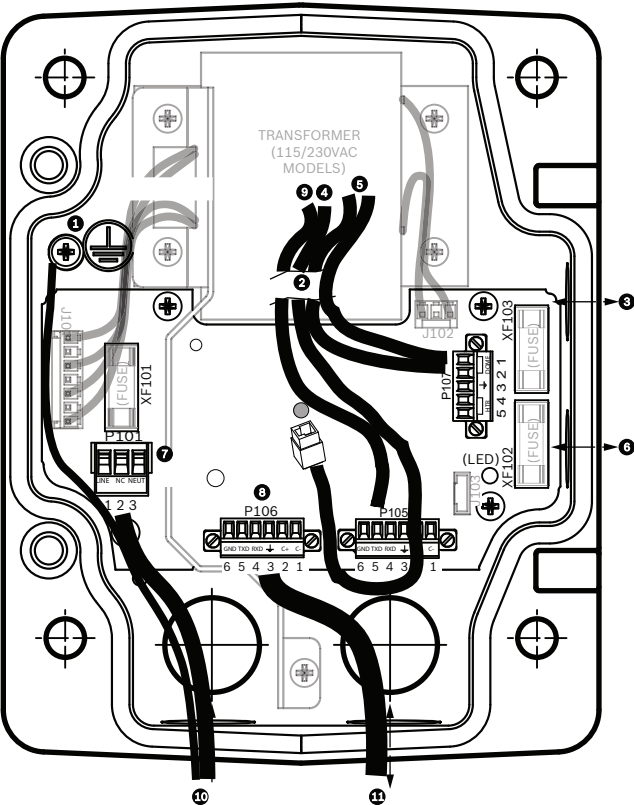
Bild 8.2: Hängearmnetzteilkasten
