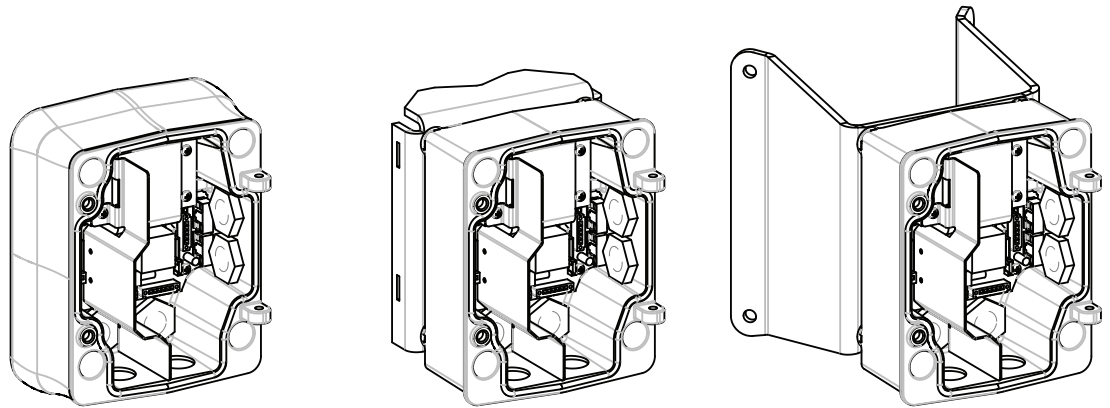
Bild 7.1: Netzteilkasten mit Wand-, Mast- und Eckenhalterung
